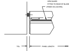
660. JAMB DETAIL
