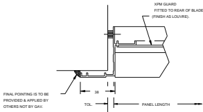
652. JAMB DETAIL
